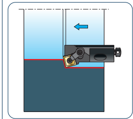
16CA..X°=45°
