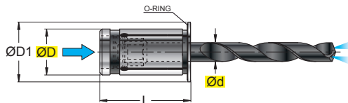
BOCCOLE DI RIDUZIONE CILINDRICHE CON GOMMA DI TENUTA PER MANDRINI IDRAULICI CYLINDRICAL REDUCTION COLLETS WITH O-RING FOR HYDRAULIC CHUCKS ZYLINDRISCHE REDUZIERBUCHSEN MIT GUMMIDICHTUNG FÜR HYDRAULISCHE WERKZEUGAUFNAHMEN DOUILLES DE RÉDUCTION CILINDRIQUES AVEC JOINT TORIQUE ETANCHE EN CAOUTCHOUC POUR MANDRINS HYDRAULIQUES
