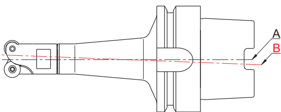
A - Asse di rotazione - Axis of rotation B - Asse geometrico - Geometric axis or barycenter
