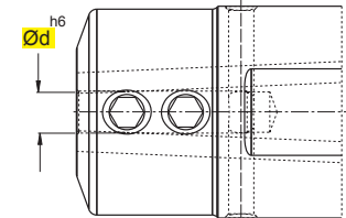
art. S100-TS-..
