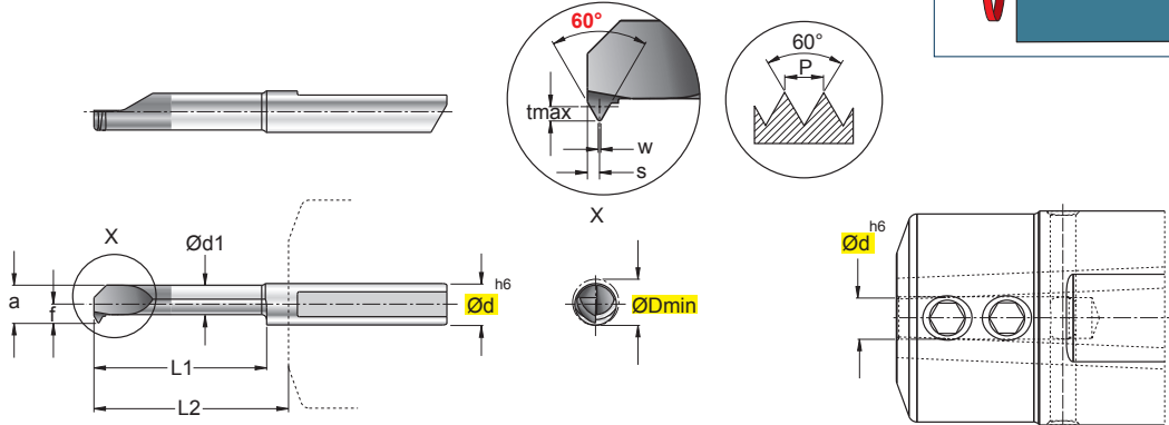
art. S100-TS-..
