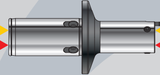
380.080.063.100 RDU.063.0...
