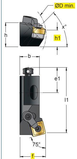
16CA..X°=45°
